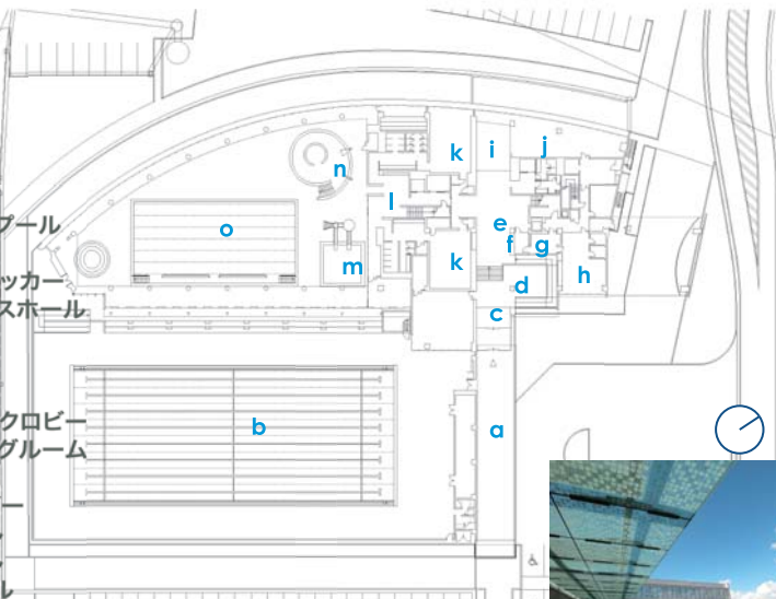
1F PLAN S=1:1500
