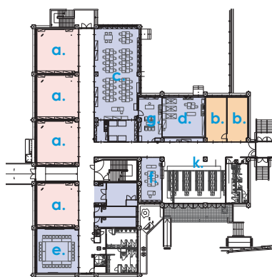
本館棟 1F PLAN S=1:1500
