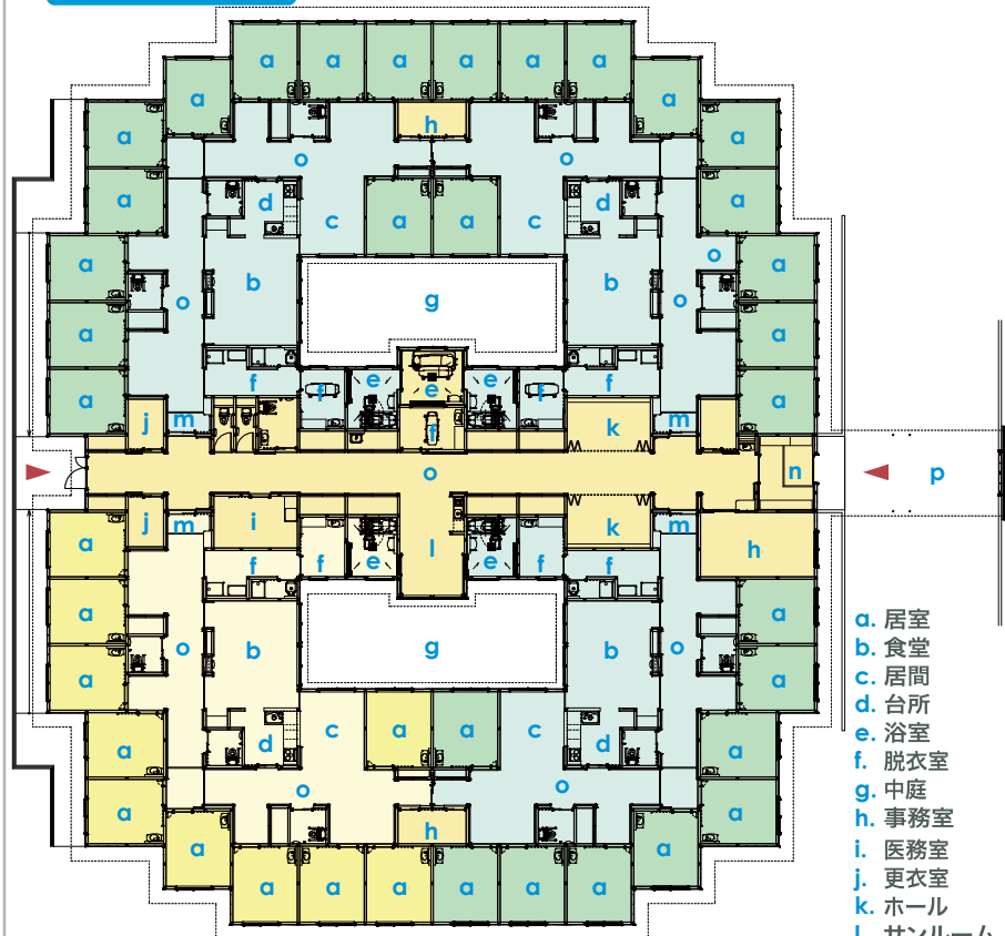
1F PLAN S=1:400
