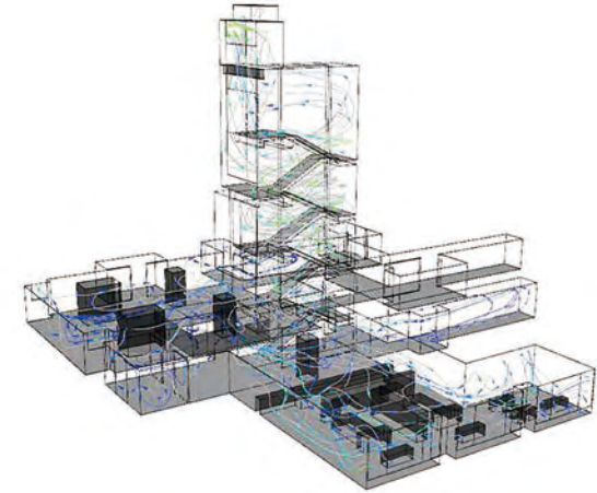
自然通風シミュレーション 春日警察署
